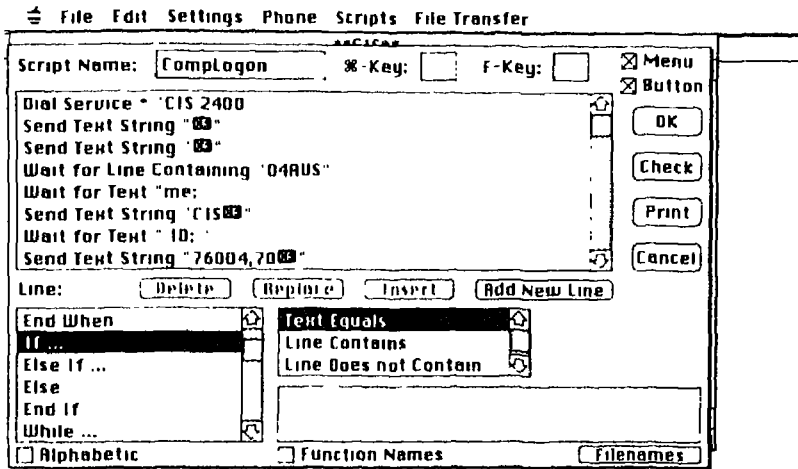
شكل (٨-١) : منقح نصوص Micro Phone II .
